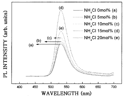
그림 3. NH 4 Cl 농도에 따른 Zn 2 SiO 4 :Mn 형광체의 PL 스펙트럼.
