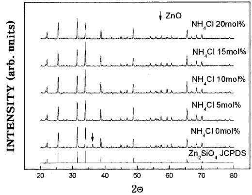
그림 2. NH 4 Cl 농도에 따른 Zn 2 SiO 4 :Mn 형광체의 XRD 패턴.
