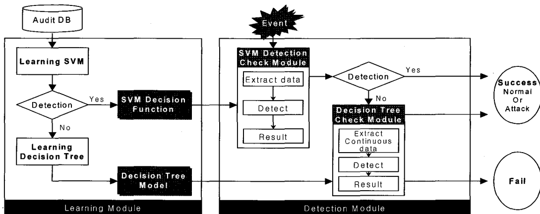
(그림 1) 제안 프레임워크
