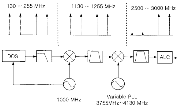
그림 3. 고속 광대역 DFS 구성도 Fig. 3. High speed wideband DFS configuration
