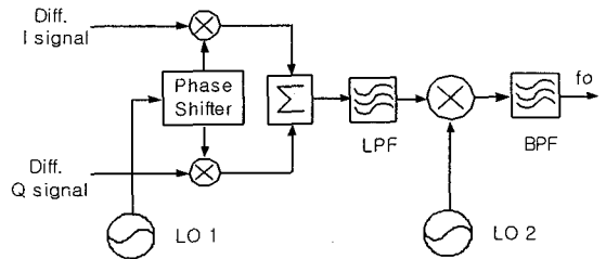
그림 1. 2개 이상의 신호 발생기를 사용한 간접 주파수 변환 구조
