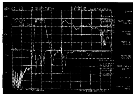
그림 4. 설계된 광대역 대역 통과 필터의 대역 특성 Fig. 4. Frequency response of designed wideband band-pass filter
