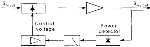
그림 5. ALC 구성도 Fig. 5. ALC configuration
