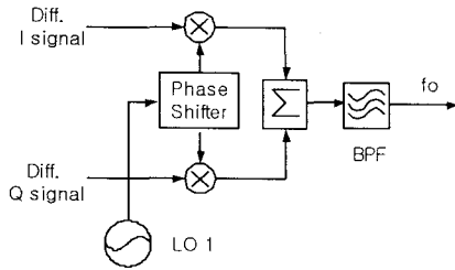
그림 2. 고속 광대역 DFS를 사용한 직접 주파수 변환 구조 Fig. 2. Direct frequency conversion scheme using high speed wideband DFS
