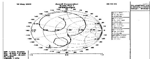
(c) 스미트 차트 데이터 (c) Smith chart data
