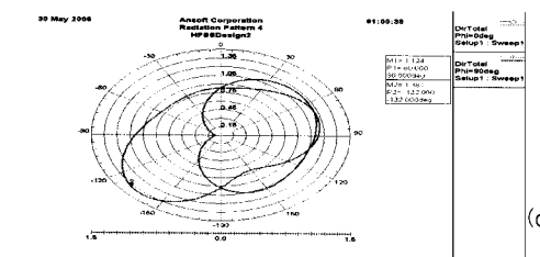
(d) U_PCS 1850MHz 대역 H/E 방사패턴 (d) H/E Radiation pattern of U_PCS 1850MHz Band
