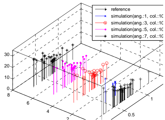
(그림 7) 방사각에 따른 ray의 impulse response
