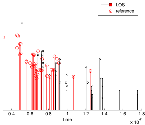
(그림 5) Ray의 impulse response (방사각 1°)
