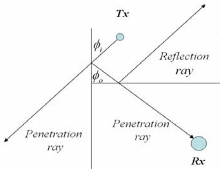
(그림 2) Ray의 반사 및 투과
