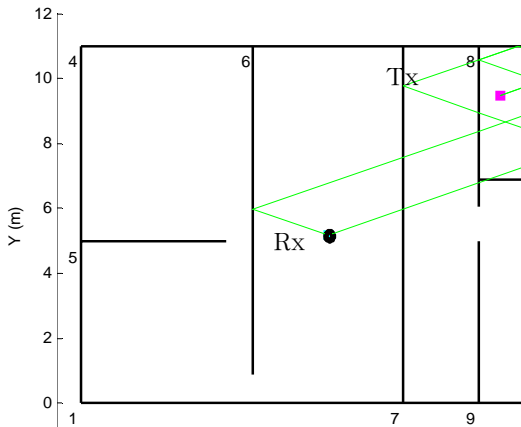
(그림 3) 다중벽면의 실내 환경
