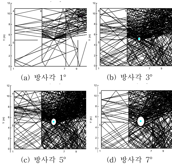
(그림 4) 방사각에 따른 ray의 경로 패턴
