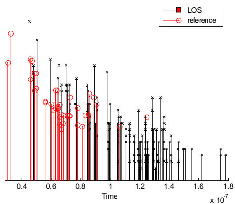
(그림 6) Ray의 impulse response (방사각 3°)
