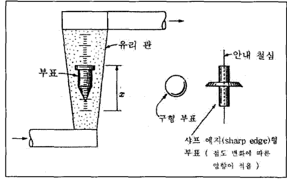
Fig. 2 면적식 유량계
