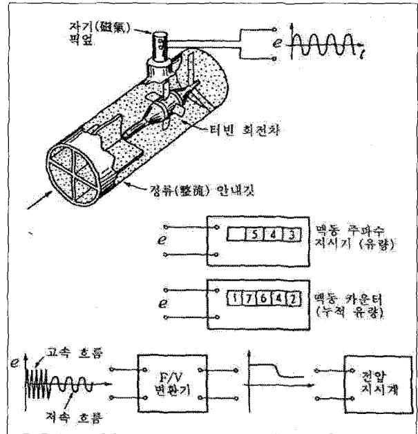
Fig. 5 터빈 미터
