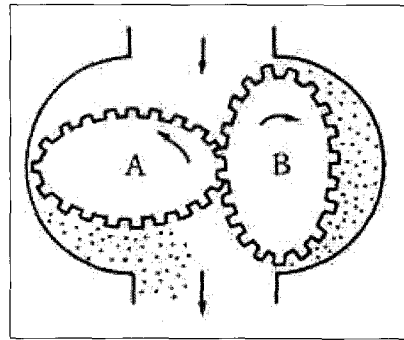
Fig. 3 오발(Oval) 유량계
