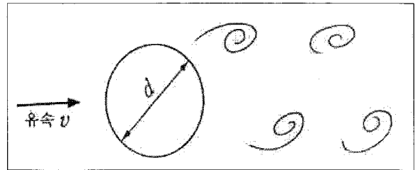
Fig. 9 Karman 渦列
