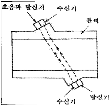
Fig. 8 관로 외부 부착형 초음파 유량계
