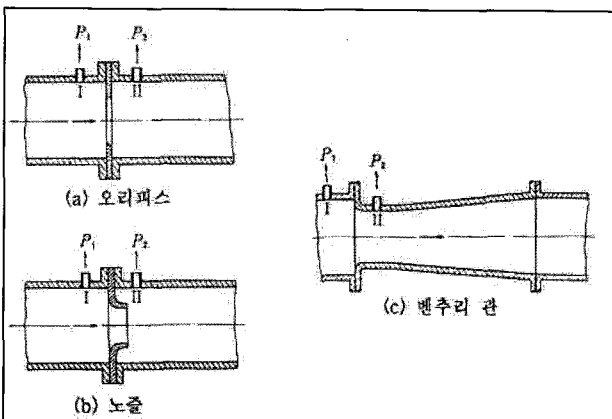
Fig. 1 차압식 유량계의 구조
