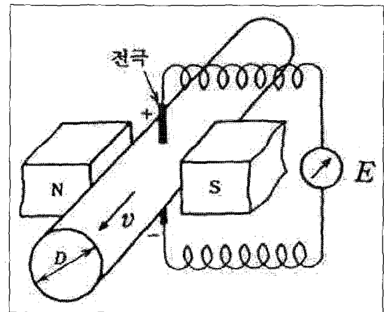
Fig. 6 電磁 유량계
