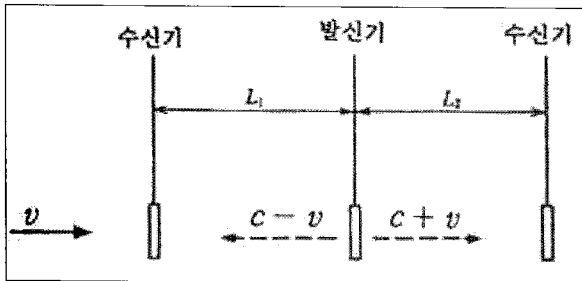
Fig. 7 초음파 유량계의 원리
