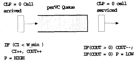
그림 3. 제안된 스케줄링 동작
