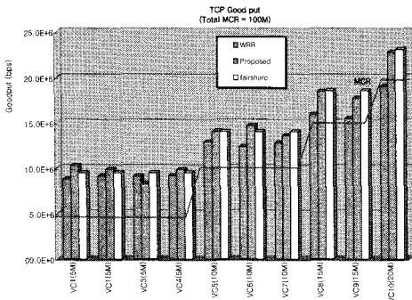
그림 7. TCP Goodput
