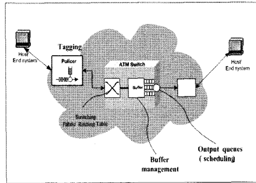
그림 1. ATM 네트워킹의 스케줄러 구조
