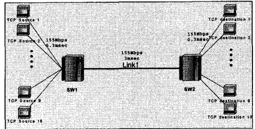
그림 6. 시뮬레이션 모델
