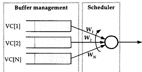
그림 2. WRR 스케줄링 구조
