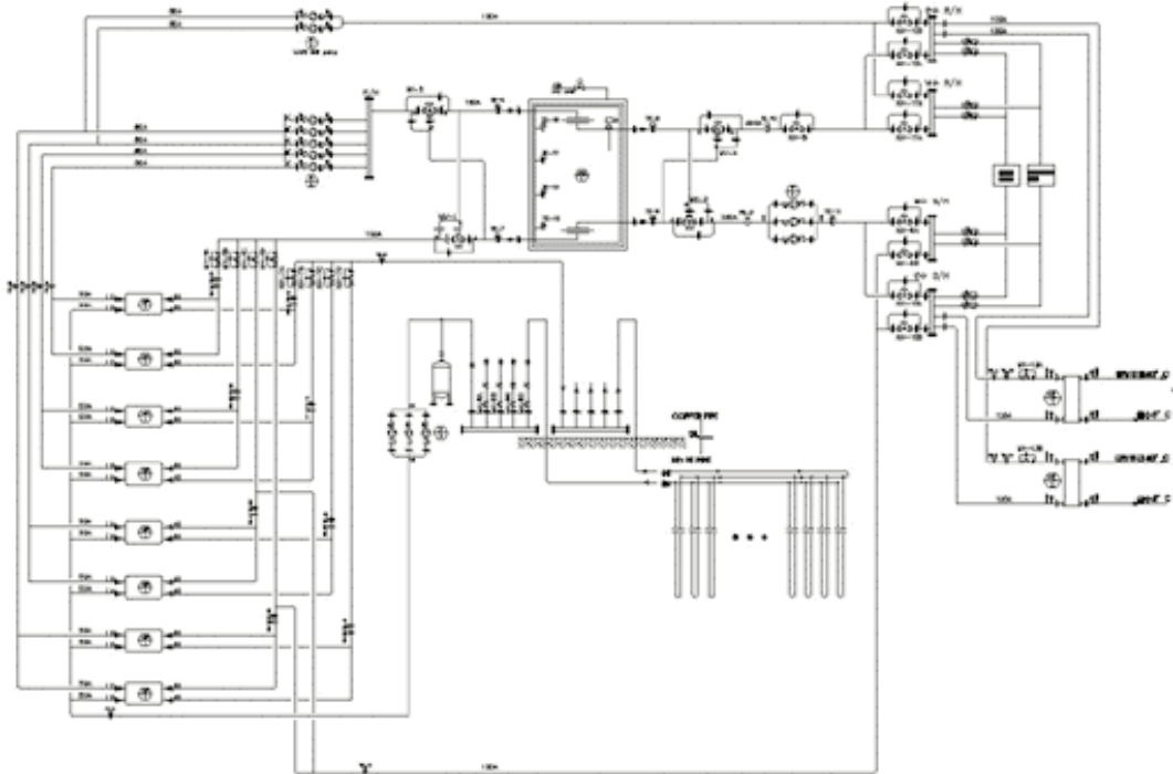
[그림 2] 지열시스템 흐름도
