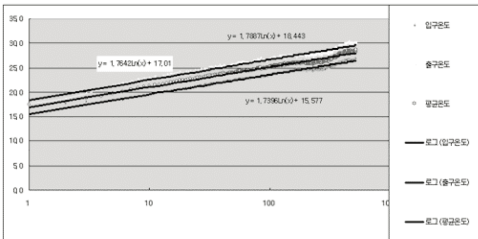
[그림 13] 지열 열전도도 테스트 데이터 그래프(창녕서드페이지)
