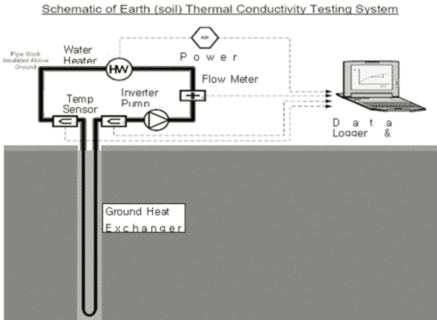
[그림 11] 지열 열전도도 테스트 개념도
