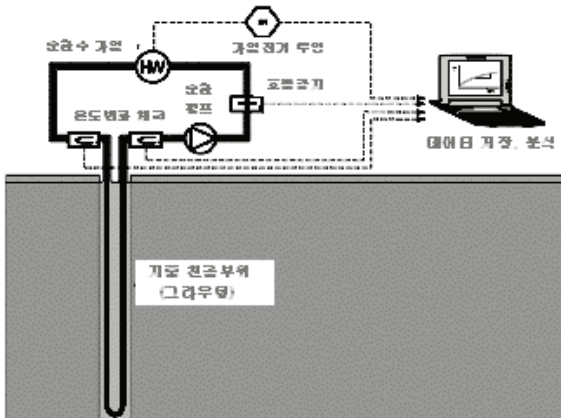
[그림 4] 지열 열전도도 개념도 및 테스트
