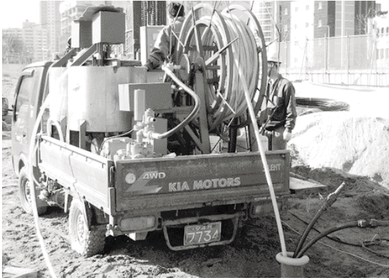
[그림 7] 지열 그라우팅
