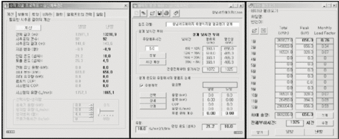
[그림 14] 지열 열교환기 설계 프로그램(GLD)
