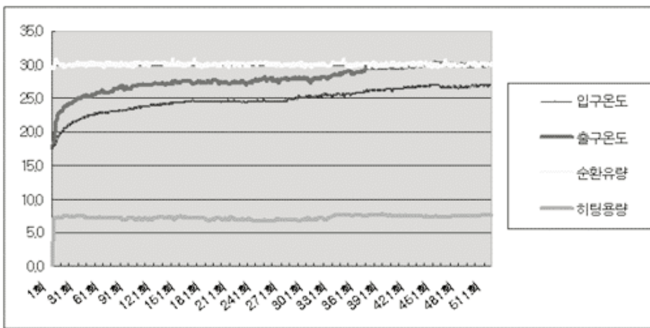
[그림 12] 지열 열전도도 테스트 데이터 그래프(창녕서드페이지)
