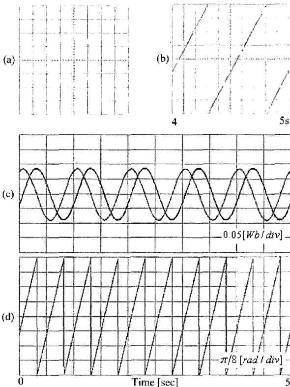
그림 7 제안된 방법으로 전류추정오차(+10 % 오프셋 전류, k_a=0.9 , k_b=0.8 )를 보상한 결과. (a) 추정된 회전자 자속의 X-Y plot. (b) (d)의 어두운 부분을 확대한 파형. (c) 추정된 회전자 자속. (d) 추정된 회전자 각위치 및 실제 회전자 각위치.
