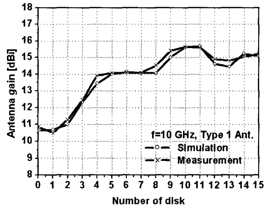
그림 13. 원형 도체 적층 수 변화에 따른 측정 및 시뮬레이션 이득 비교
