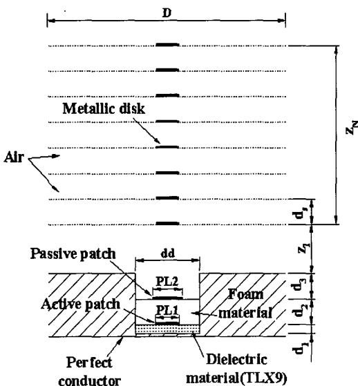
그림 1. 고이득 성형 빔 안테나 구조 Fig. 1. High gain shaped-beam antenna structure.
