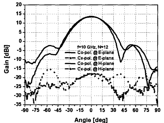
그림. 11. Type 2 안테나의 N=12 에서 측정된 방사 패턴 성능
