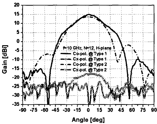
(b) H-plane
