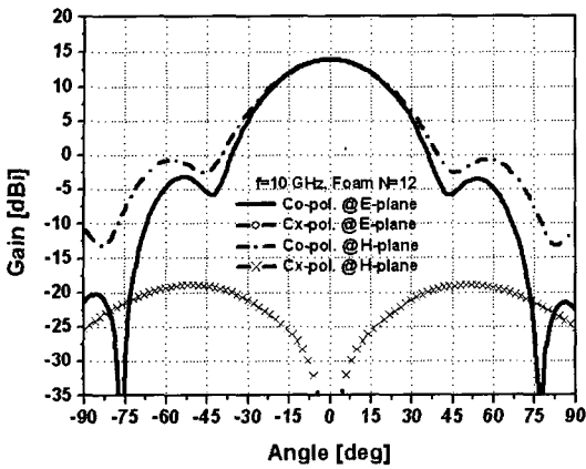
그림 5. Type 2 안테나의 시뮬레이션 방사 패턴 성능(N=12) Fig. 5. Simulated radiation pattern performance of Type 2 antenna(N=12).
