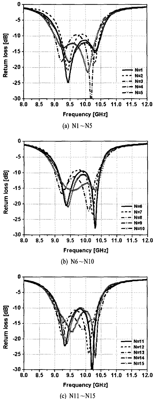
그림 8. Type 1 안테나의 측정된 입력 반사 손실 성능 Fig. 8. Measured input return loss performance of Type 1 antenna.
