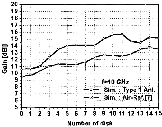
그림 6. 원형 도체 적층 수 변화에 따른 시뮬레이션 이득 비교 Fig. 6. Antenna gain comparison simulated by the variations of metallic disk stack number.
