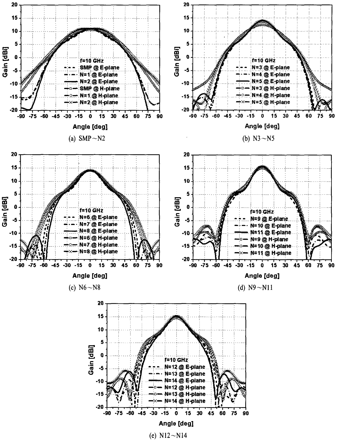
그림 4. Type 1 안테나의 시뮬레이션 방사 패턴 성능 Fig. 4. Simulated radiation pattern performance of Type 1 antenna.
