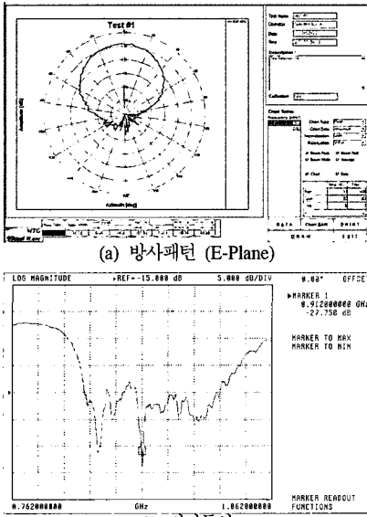
그림 13. LHCP 안테나의 방사패턴과 반사특성
