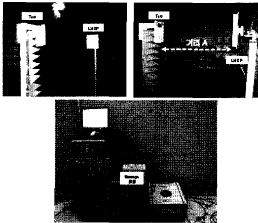
그림 17. 테스트 환경사진
