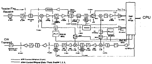
그림 7. RF Shower 시스템 블록도
