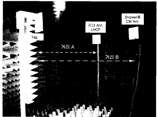
그림 19. 실험 안테나 배치도
