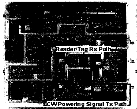
그림 10. XCVR(Transceiver) 설계사진
