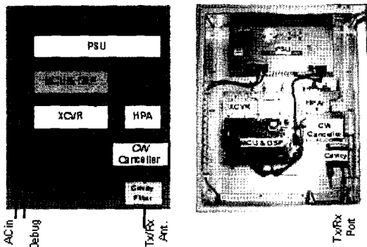
그림 8. RF Shower 시스템 구현
