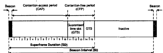
그림 1. 비콘 구간과 슈퍼프레임 구간
