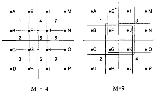
그림 2. 제안된 Reduced Complexity QRM-MLD기법의 첫 번째 step의 송신신호 후보군을 선택하는 방법 Fig. 2. Candidate set selection method in the first step of the reduced complexity QRM-MLD proposed in the paper
