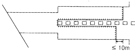
그림 1. 동시굴착공법(2-Arch 터널)
