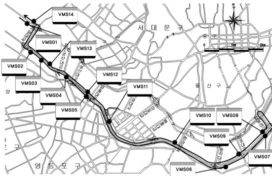
<그림 3> 1차 현장조사 VMS 설치 위치도
