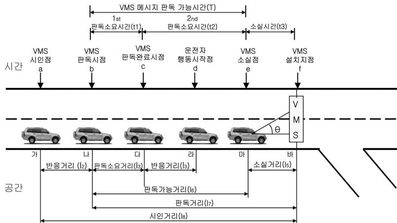
<그림 1> VMS 판독거리 개념도
