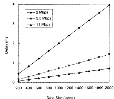
그림 15. CR 비콘 평균 전송 지연
