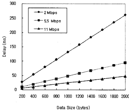
그림 18. 릴레이 지연
