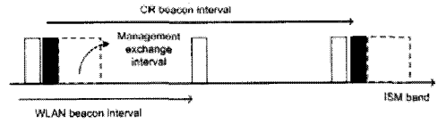
그림 3. WLAN 비콘과 CR 비콘 운영
