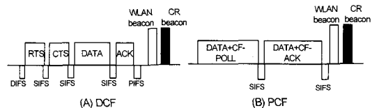
그림 11. CR 비콘 전송 예
