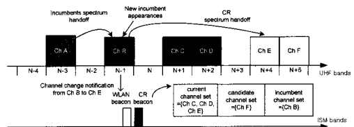
그림 9. 핸드오버 예
