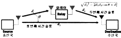
그림 1. 이중 홉 DF 릴레이 시스템
