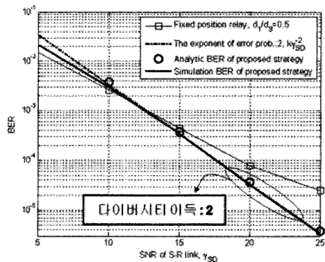
그림 2. \gamma_{SD} = \gamma_{RD} 인 경우, 고정된 위치의 릴레이와 제안된 릴레이 위치 기법의 성능 비교 ( \alpha = 4 )
