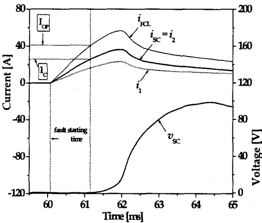
그림 7. 병렬연결시 초기사고전류제한 특성 Fig. 7. Initial fault current limiting characteristics of SFCL in case of parallel connection of two coils
