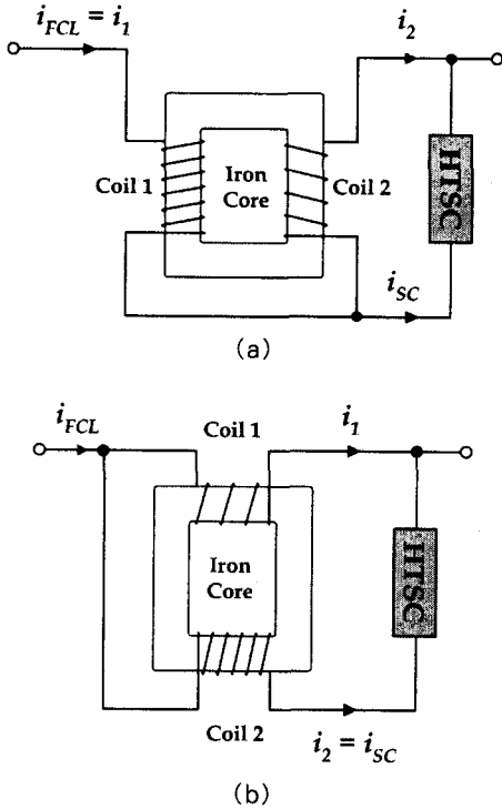
그림 1. 코일의 자기결합을 이용한 초전도 사고전류 제한기의 구조 (a) 직렬연결형 (b) 병렬연결형 Fig. 1. Structure of superconducting fault current limiter (SFCL) using magnetic coupling of two coils (a) Series connection type (b) Parallel connection type
