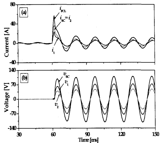
그림 5. 병렬연결시 사고전류제한 특성 (a) 전류파형 (b) 전압파형
