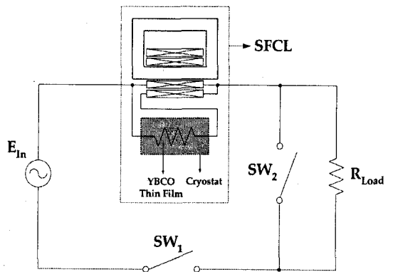
그림 3. 초전도 사고전류제한기의 모의실험회로도 Fig. 3. Experimental circuit of SFCL
