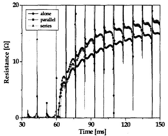
그림 8. 초전도 소자의 저항곡선 Fig. 8. Resistance curves of HTSC element
