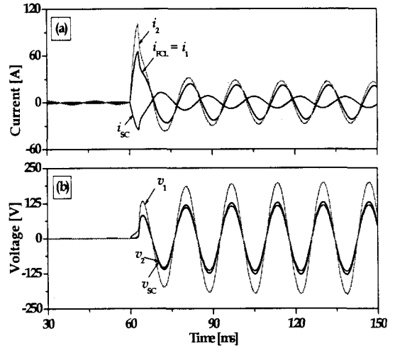
그림 4. 직렬연결시 사고전류제한 특성 (a) 전류파형 (b) 전압파형
