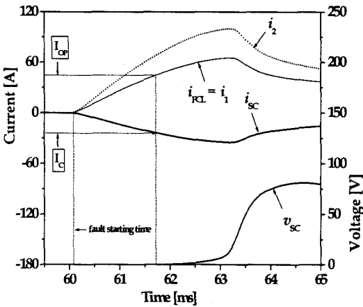
그림 6. 직렬연결시 초기사고전류제한 특성 Fig. 6. Initial fault current limiting characteristics of SFCL in case of series connection of two coils
