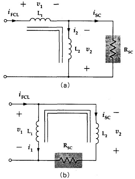
그림 2. 코일의 자기결합을 이용한 초전도 사고전류 제한기의 등가회로 (a) 직렬연결형 (b) 병렬연결형 Fig. 2. Equivalent circuit of SFCL using magnetic coupling of two coils (a) Series connection type (b) Parallel connection type
