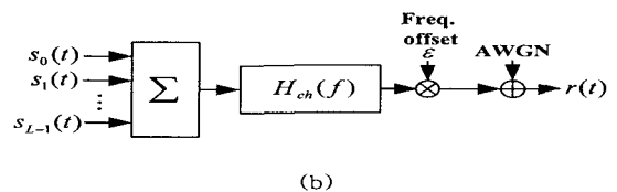
그림 2. 전송 채널 구조((a)상향 링크, (b)하향 링크). Fig.2 Channel structure((a)uplink, (b)downlink).
