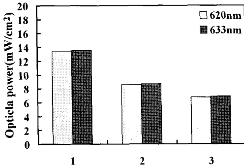
그림 3. 광 출력 특성. Fig. 3. Characteristics of optical power of experiment.
