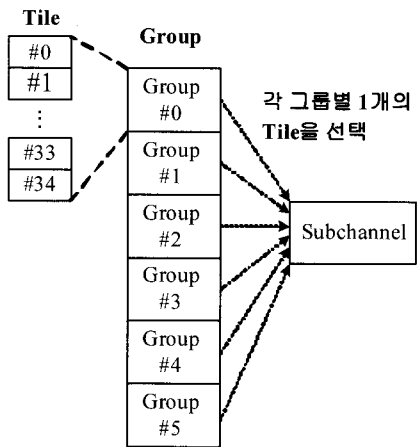
그림 2. WiBro 상향링크 부채널 할당 과정
