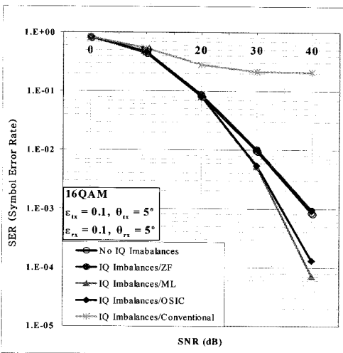
그림 6. 송수신 이득 불균형 0.1, 위상 불균형 5°인 경우 16QAM에서의 SER 성능
