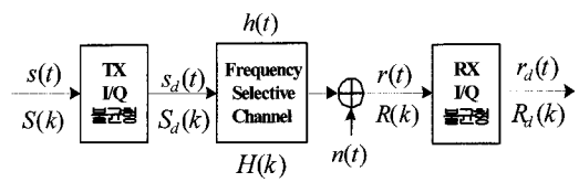
그림 3. 송수신 I/Q 불균형과 다중경로 채널 응답이 결합된 기저대역 시스템의 등가모델
