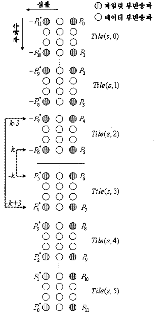
그림 4. 새로 제안된 새로운 부채널 할당 방식
