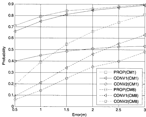
그림 11. 각 기법 별 SOP에 따른 TOA 오차 성능에 대한 비교(SNR = 10 dB, SOP = 4)
