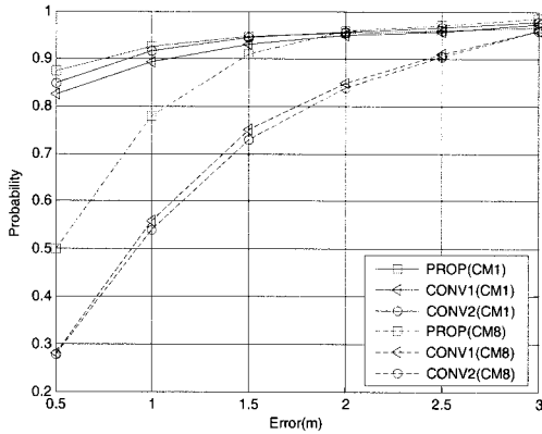
그림 10. 각 기법 별 SOP에 따른 TOA 오차 성능에 대한 비교(SNR = 10 dB, SOP = 0)
