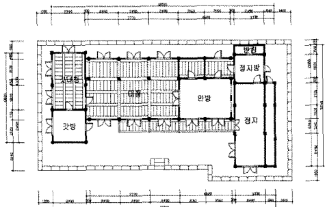
<그림 13> 양동호 가옥 안채 평면도
