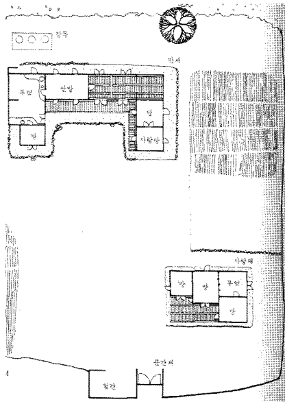
<그림 8> 여산송씨 종가 배치도하 (1986년 필자실측)
