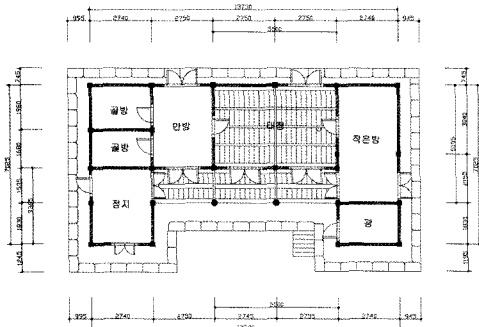
<그림 11> 김선기 가옥 안채 평면도 (2006년 필자 실측)
