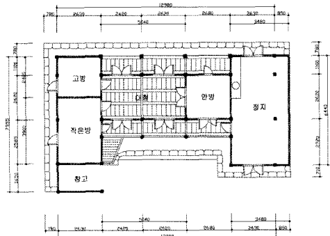
<그림 12> 정학남 가옥 안채 평면도 (2006년 필자 실측)
