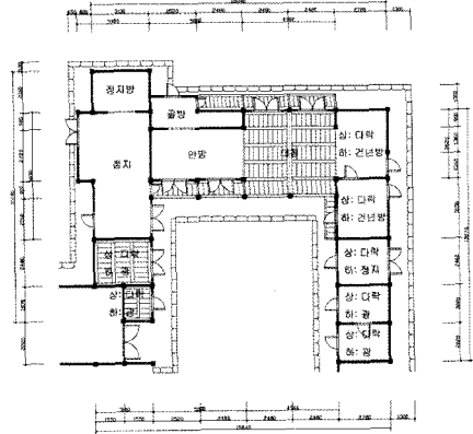
<그림7> 운조루 안채 평면도
