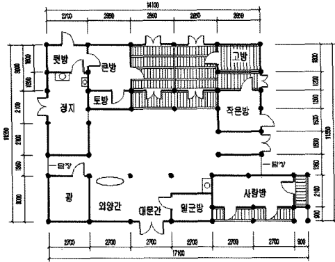
<그림5> 필자가 치수선을 넣어 새로 그린 위성렬 가옥 평면도
