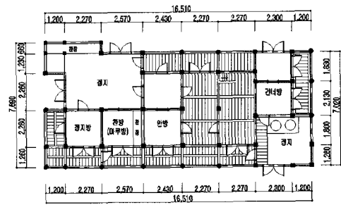
<그림 16> 나상열 가옥 안채 평면도
