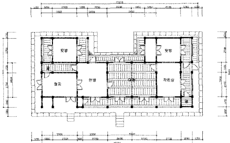
<그림 3> 이금재가옥 안채 평면도 (2006년 필자실측)
