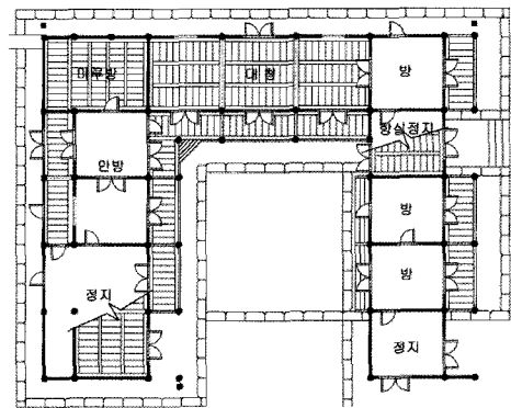
<그림 10> 윤두서 가옥 안채 평면도 (2006년 필자 실측)
