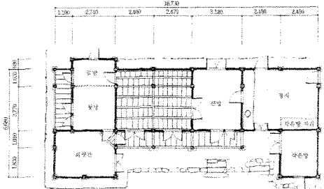
<그림 14> 정무경 가옥 안채 평면도 (1993년 필자 실측)
