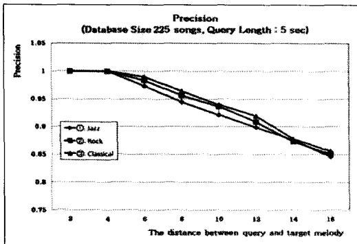
그림 34 질의의 부정확한 정도에 따른 장르별 정밀도
