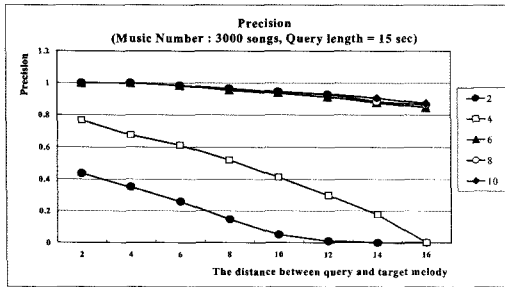
그림 22 FMLT값에 따른 정밀도 비교
