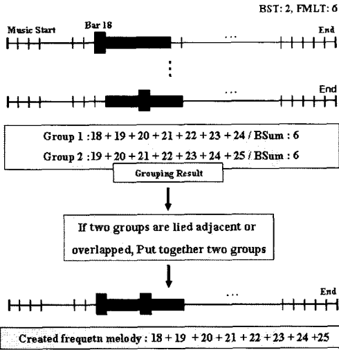
그림 9 중복된 멜로디 처리
