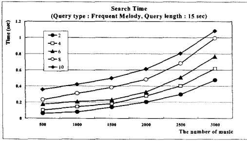
그림 20 FMLT의 값에 따른 빈번 멜로디 인덱스의 검색 시간
