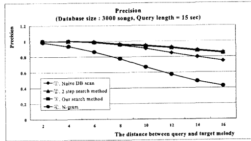
그림 30 질의의 부정확한 정도에 따른 정밀도
