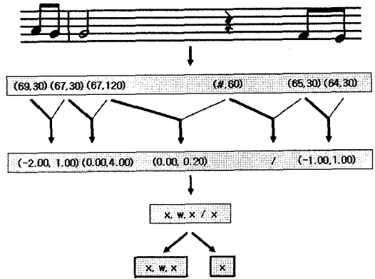
그림 11 멜로디를 한 박자 이상의 쉼표로 나누는 과정
