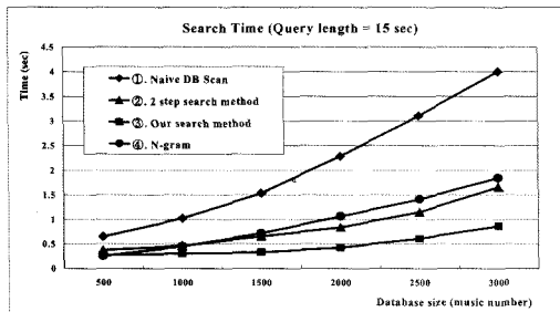
그림 27 데이터베이스 크기에 따른 검색 시간
