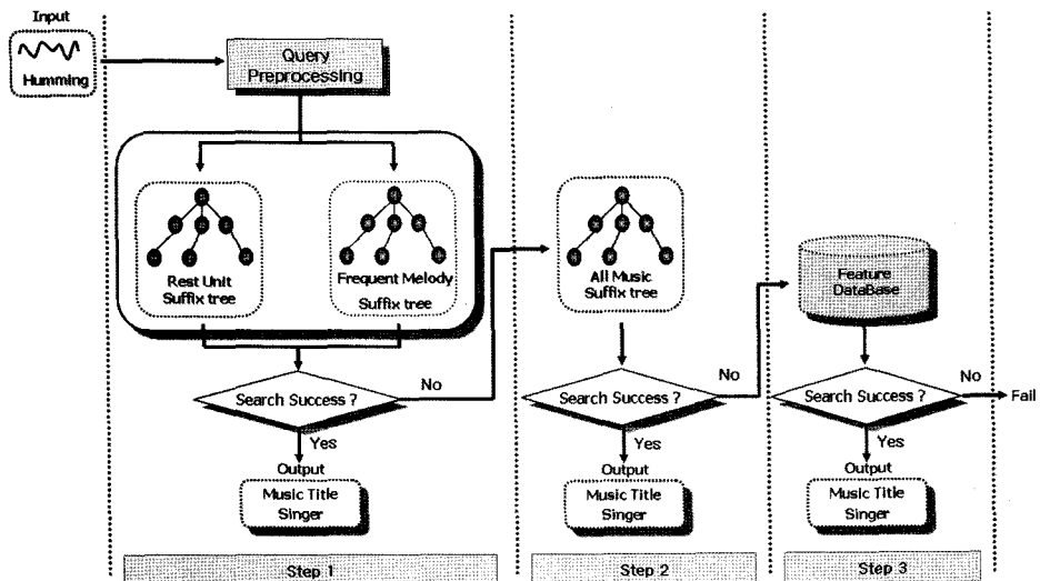
그림 13 질의 처리 과정
