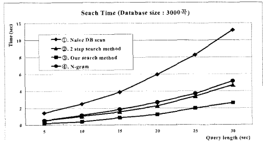
그림 28 질의 길이에 따른 검색시간
