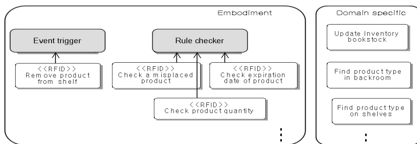
(그림 5) 도메인 액티비티 도출과정
