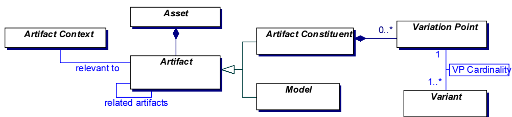
(그림 1) 소프트웨어 프로덕트 라인 자산 메타모델
