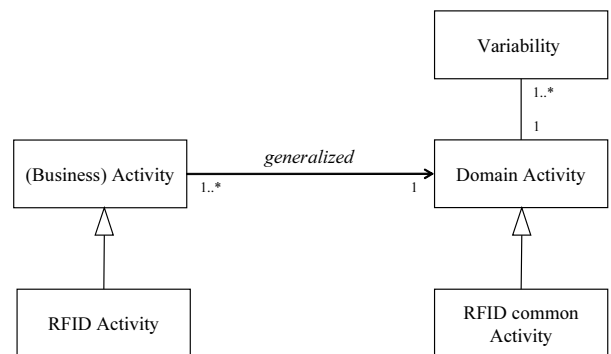
(그림 3) RFID PLA를 위한 액티비티 분류
