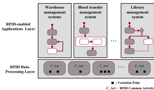
(그림 2) RFID 애플리케이션을 위한 2-계층 구조
