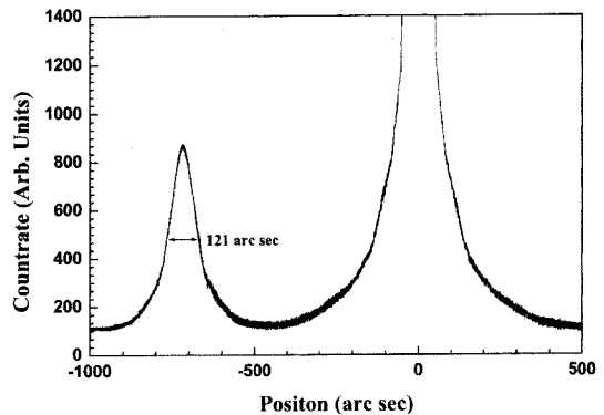
그림 2. \text{AgInS}_2 박막의 이중 결정 X-선 요동 곡선
