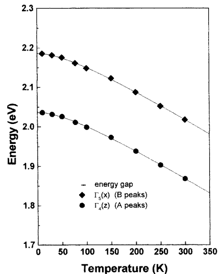
그림 4. 온도의 함수로서 나타낸 광전류 에너지와 에너지 밴드 갭
