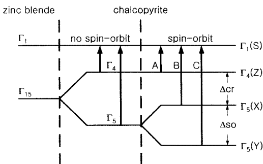
그림 5. Selection rule에 따른 \Gamma point에서의 chalcopyrite \text{AgInS}_2 박막의 에너지 밴드 구조 Fig. 5. Energy band structure of the chalcopyrite \text{AgInS}_2 at the \Gamma point according to the selection rule.
