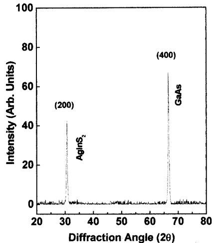
그림 1. GaAs 기판 위에 성장된 \text{AgInS}_2 박막의 X-선 회절 무늬
