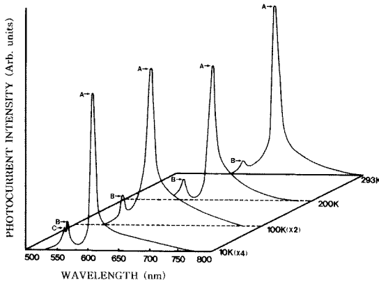
그림 3. 여러 온도에서 측정된 AgInS 2 박막의 광전류 스펙트럼
