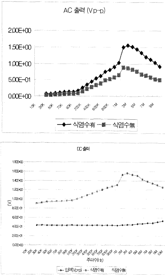
그림 7. 주파수 특성 Fig. 7. Frequency characteristics.
