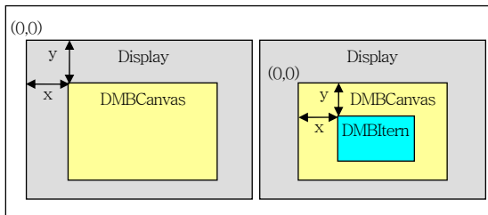
(그림 5) DMBCanvas 및 DMBItem 좌표계
