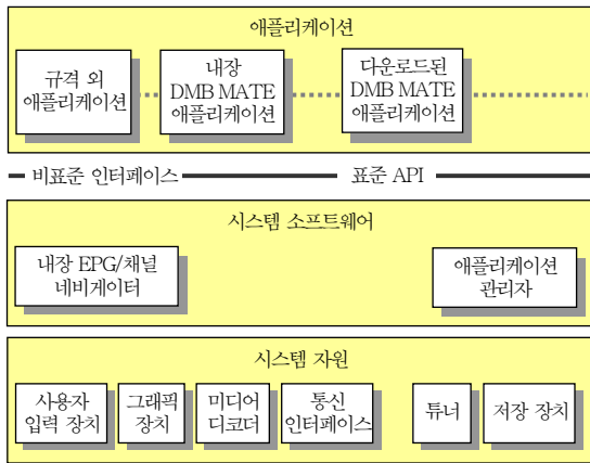
(그림 1) 기본 수신기 모델
