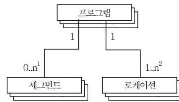
(그림 10) 스케줄 정보를 구성하는 서비스 객체간의 관계도
