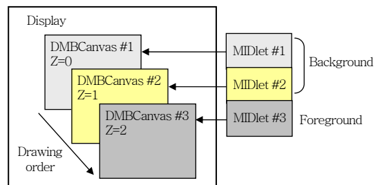
(그림 4) Z Order 관리 방식
