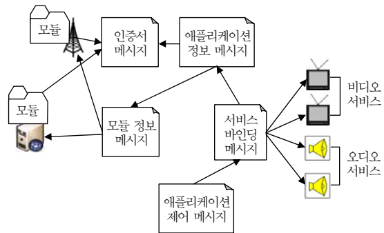
(그림 8) 시그널링 구조
