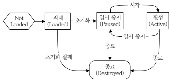
(그림 6) 애플리케이션 실행 주기
