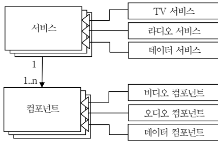
(그림 9) 서비스 목록을 구성하는 서비스 객체간의 관계도
