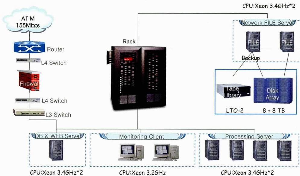
국제데이터센터 시스템 구성도
