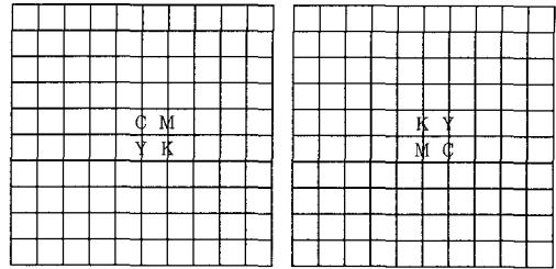
(a) 이진 데이터 1 (b) 이진 데이터 0 그림 7. 하프톤 셀과 스폿 (a) binary 1 (b) binary 0 Fig. 7. A halftone cell and a spot.
