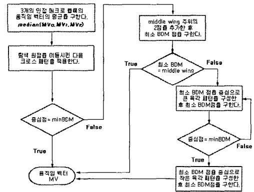
그림 8. 제안하는 알고리즘의 탐색 흐름도 Fig. 8 Search Flow of the proposed Algorithm
