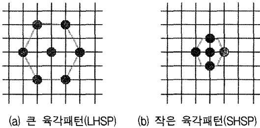
그림 2. 육각패턴 탐색 알고리즘의 탐색 패턴 Fig. 2 Search patterns used in the HEXBS
