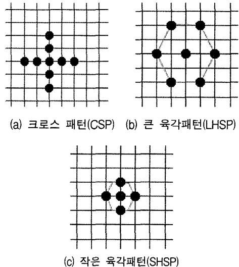
그림 4. 크로스-육각패턴 탐색 알고리즘의 탐색 패턴 Fig. 4 Search patterns used in the CHS
