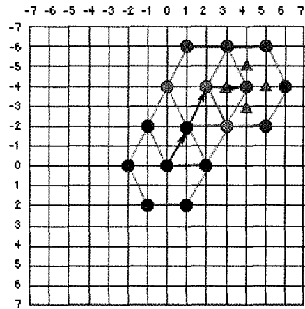
그림 3. 육각패턴 탐색 알고리즘의 탐색 경로 Fig. 3 Search path of the HEXBS
