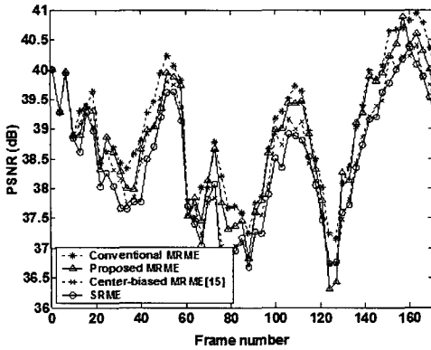
그림 4. 테스트 영상 QCIF 'Car phone' 에 대한 PSNR 그래프 (GOP=IPPP., 64kbps, 프레임율=10Hz). Fig. 4. PSNR for a QCIF 'Car phone' sequence, (GOP=IPPP., 64kbps, Frame rate=10Hz).
