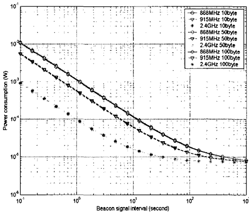
그림 8. 비콘 신호 주기 및 down-link 데이터 크기에 따른 868 MHz, 915 MHz, 2.4 GHz 주파수 대역 전력소모량 (up data = 50 byte, N = 10)
