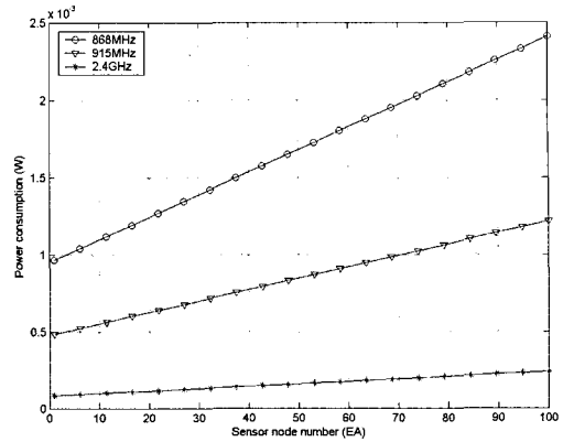
그림 6. 센서 노드 수에 따른 868 MHz, 915 MHz, 2.4 GHz 주파수 대역 전력소모량 ( T_W = 1 초, up, down data = 50 byte)
