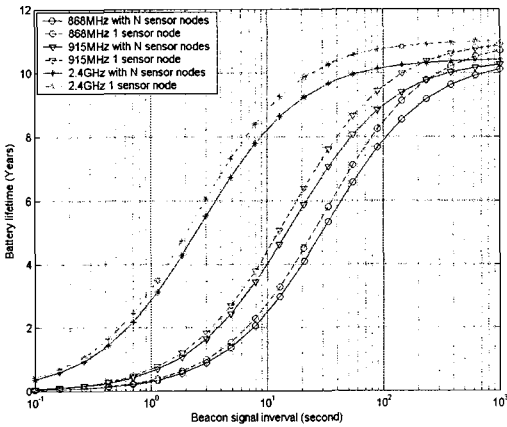
그림 5. 비콘 신호 주기에 따른 868 MHz, 915 MHz, 2.4 GHz 주파수 대역 배터리 사용시간 (up, down data = 50 byte, N = 10)
