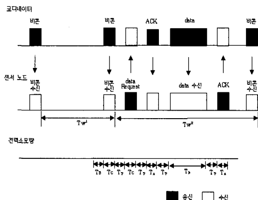
그림 1. IEEE 802.15.4 down-link 모델 및 전력소모량
