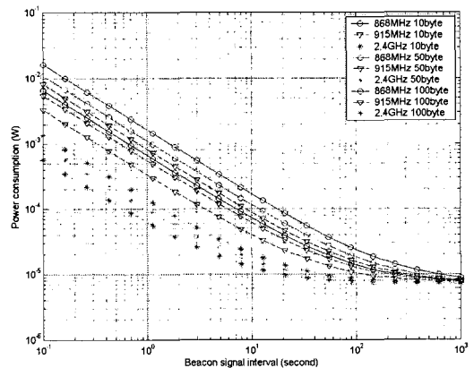
그림 7. 비콘 신호 주기 및 up-link 데이터 크기에 따른 868 MHz, 915 MHz, 2.4 GHz 주파수 대역 전력소모량 (down data = 50 byte, N = 10)
