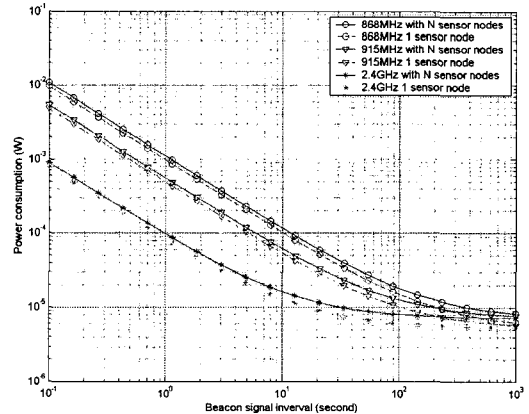
그림 4. 비콘 신호 주기에 따른 868 MHz, 915 MHz, 2.4 GHz 주파수 대역 전력소모량 (up, down data = 50 byte, N = 10)
