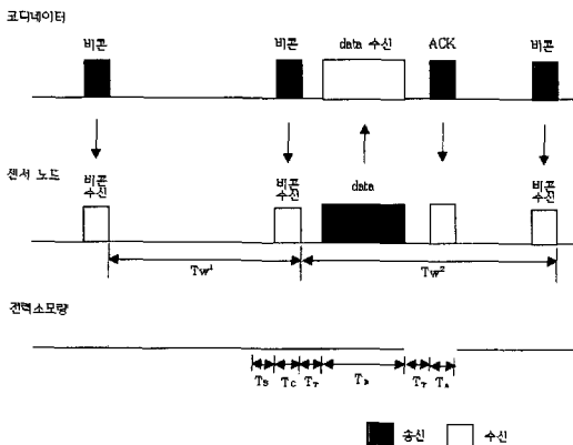
그림 2. IEEE 802.15.4 up-link 모델 및 전력소모량
