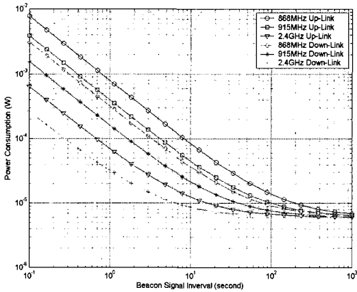
그림 3. 비콘 신호 주기에 따른 868 MHz, 915 MHz, 2.4 GHz down-link 및 up-link 전력소모량 (up, down data = 50 byte, N = 10)
