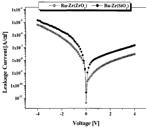
그림 4. 700 °C 급속 열처리 이후 MOS 커패시터의 게이트 누설 전류. Fig. 4. Leakage current of MOS capacitor after 700 °C rapid thermal annealing.
