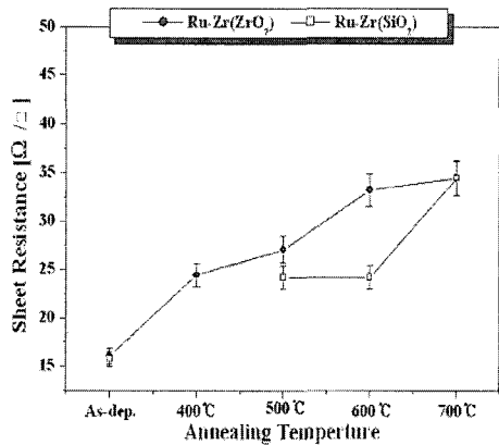
그림 5. 급속 열처리 이후의 면저항 변화. Fig. 5. The change of sheet resistance after rapid thermal annealing.
