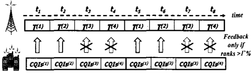
그림 3. 제안하는 TCP-OFB 방식의 개념도(G=4, Γ=50%)
