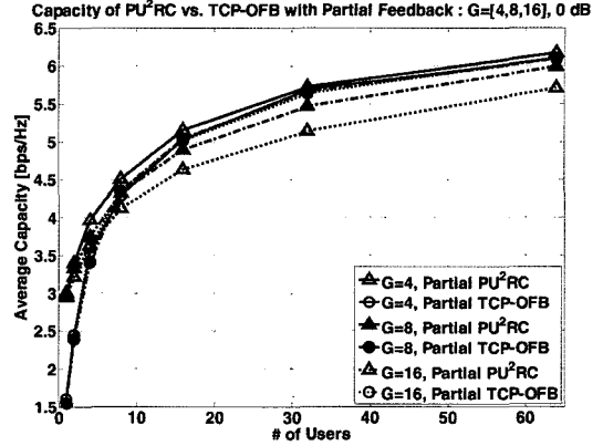
그림 4. 제안하는 TCP-OFB의 채널용량 성능(Partial Feedback 채택, G=[4,8,16])
