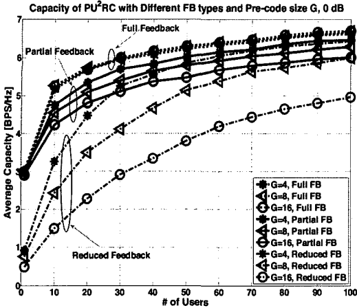
그림 2. Feedback 방식에 따른 기존 PU²RC의 채널용량 성능(코드북 크기 G=[4,8,16], SNR=0 dB)
