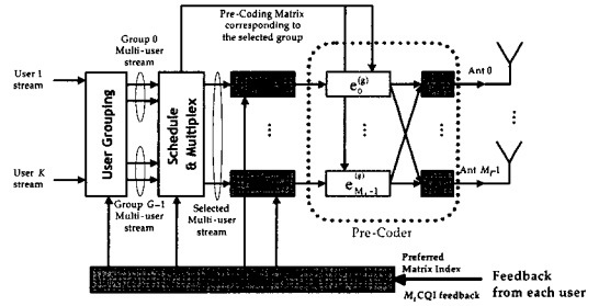
그림 1. 다중사용자 다중 입출력을 위한 PU 2 RC 시스템의 송신단
