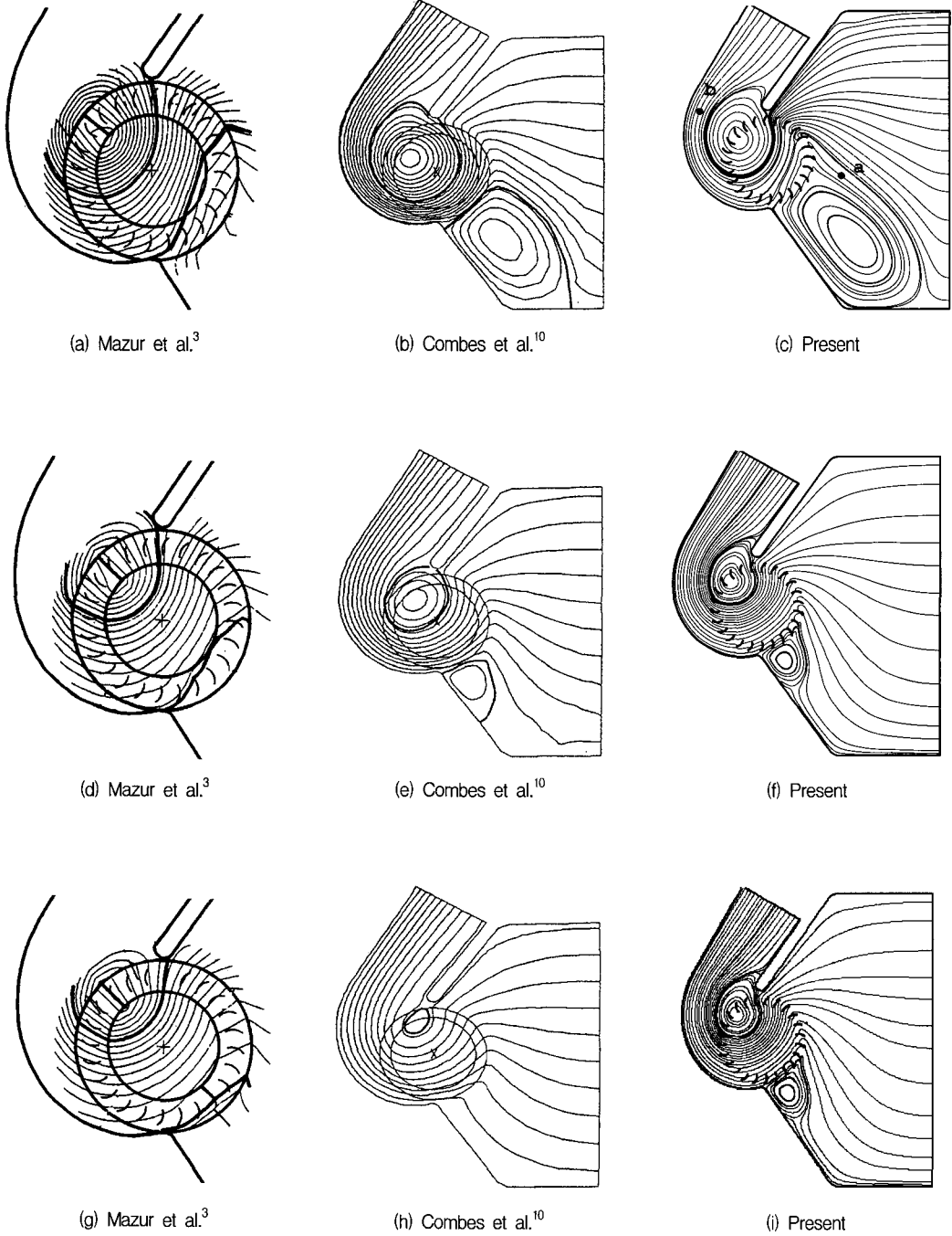
Fig. 4 Comparison of streamlines. (a)~(c):case 1, (d)~(f):case 2, (g)~(i):case3
