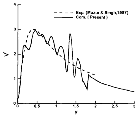
(d) Absolute velocity variation
