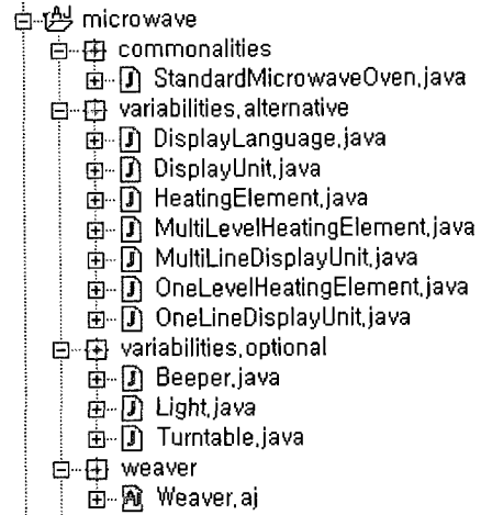
(그림 10) 클래스 구조
