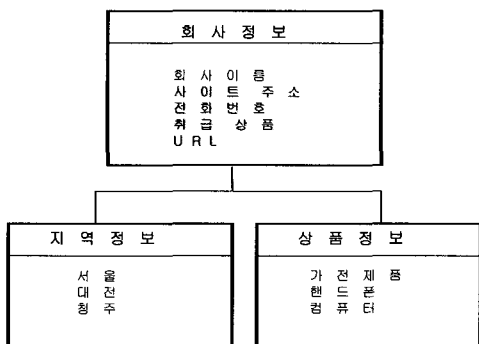
(그림 6) 쇼핑 사이트의 기본 정보 검색을 위한 온톨로지 도메인 설계
