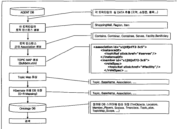
(그림 9) 온톨로지 자동 생성 과정
