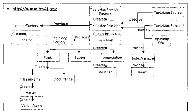
(그림 8) TM4J의 계층적 클래스도
