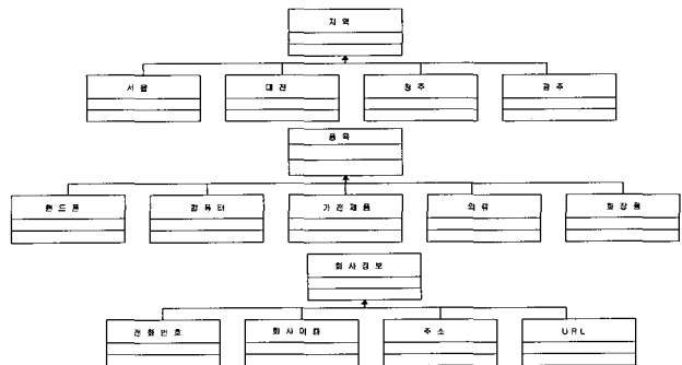
(그림 4) 토픽에 대한 클래스 구조
