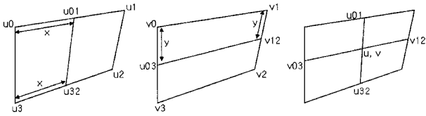
(그림 3) 역 양선형 변형을 이용한 좌표결정
