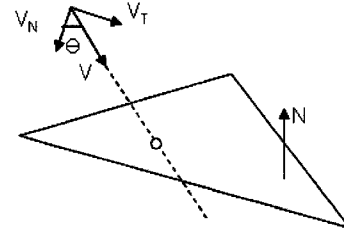
(그림 15) 충돌 상황
