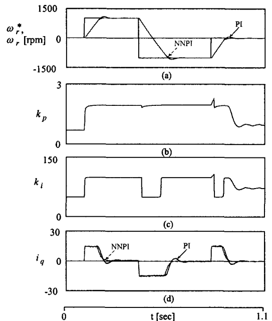
그림 9. 정·역회전 운전에 대한 응답특성 비교 Fig. 9. The comparison response characteristics with forward and reverse operation
