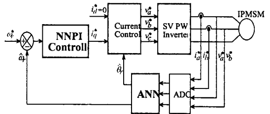
그림 6. 제시한 IPMSM의 드라이브 시스템 Fig. 6. Proposed Drive system of IPMSM
