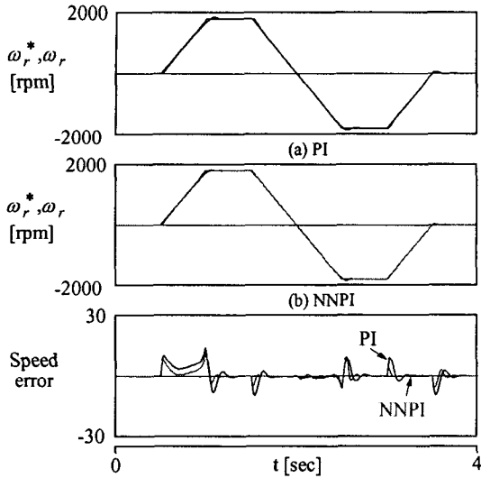
그림 13. 4상한 운전에 대한 응답특성 비교 [ J = 3J_n ] Fig. 13. The comparison of response characteristics with quadrant operation [ J = 3J_n ]
