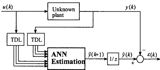
그림 5. ANN을 이용한 시스템 추정 Fig. 5. System estimation using ANN
