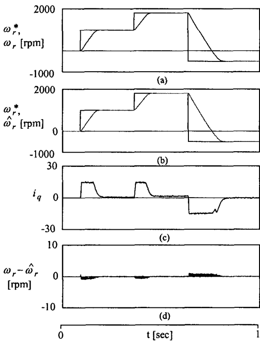
그림 14. 스텝 지령속도 변화 따른 속도 추정 Fig. 14. Speed estimation with step command speed change
