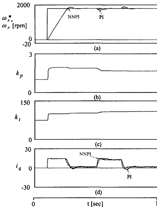
그림 7. PI와 NNPI 제어기의 응답특성의 비교 Fig. 7. The comparison of response characteristics with PI and NNPI controller
