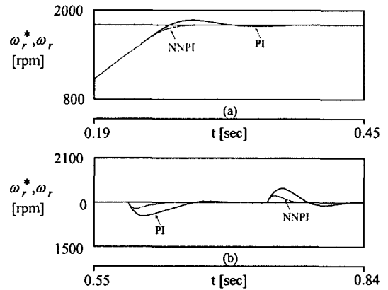
그림 8. PI와 NNPI 제어기의 응답특성의 비교 Fig. 8. The comparison of response characteristics with PI and NNPI controller
