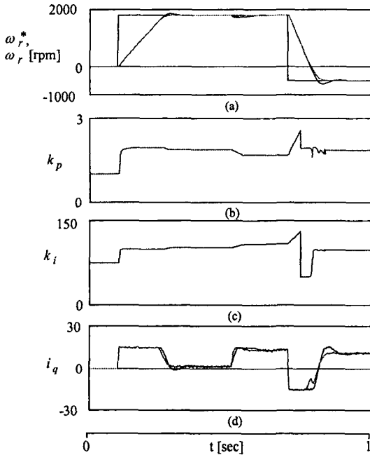
그림 10. 속도와 부하의 변화에 대한 응답특성 비교 Fig. 10. The comparison of response characteristics with speed and load torque
