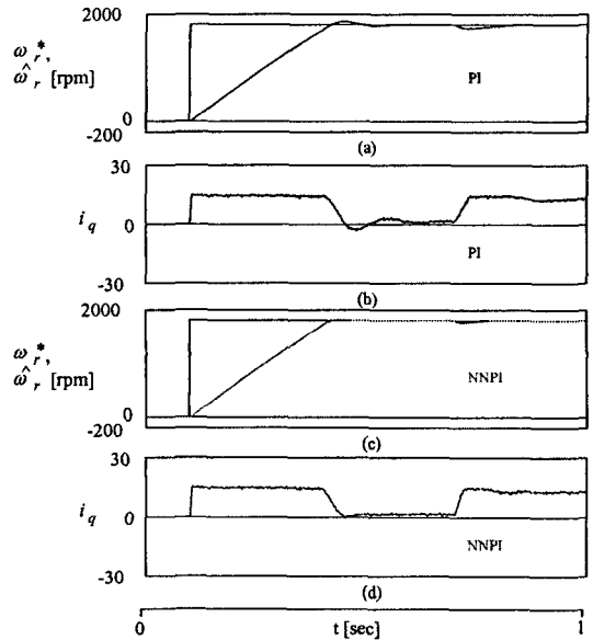
그림 11. 속도와 부하의 변화에 대한 응답특성 비교 [ J = 2J_n ] Fig. 11. The comparison of response characteristics with speed and load torque [ J = 2J_n ]
