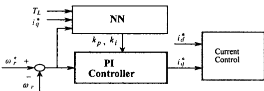
그림 2. NNPI 제어기 Fig. 2. NNPI controller
