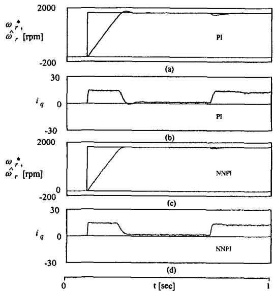
그림 12. 속도와 부하의 변화에 대한 응답특성 비교 [ R = 2R_n ] Fig. 12. The comparison of response characteristics with speed and load torque [ R = 2R_n ]
