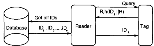
그림 2. 랜덤 해쉬 락
