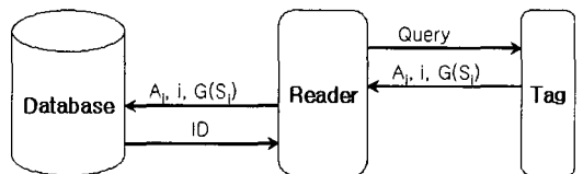
그림 3. 해쉬 체인 프로토콜
