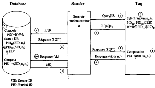
그림 4. 제안 프로토콜
