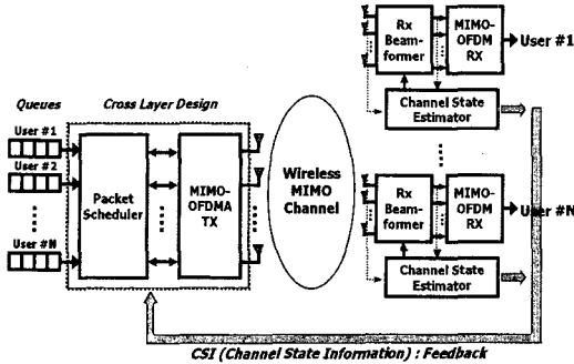
그림 1. MIMO-OFDM 다중 사용자 시스템 구조
