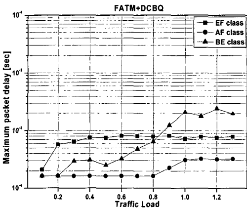
그림 11. FATM+DCBQ 큐 스케줄링 방식의 각 클래스별 최대 패킷 전송 지연
