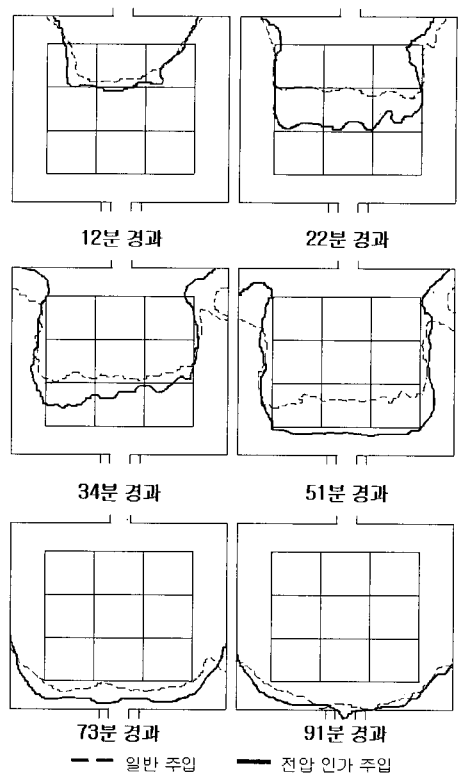
그림 5. 수직 배향 셀의 시간에 따른 액정이 주입된 영역.
