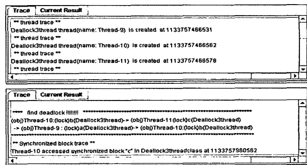
(그림 9) 데드락 발견
