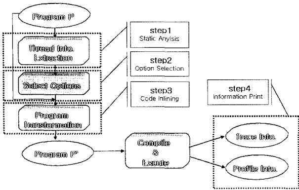
(그림 3) 시스템 구조
