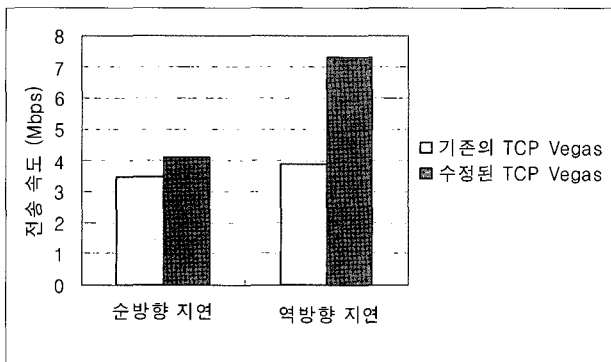
(그림 9) 순방향, 역방향 지연에 따른 초당 전송 속도 비교
