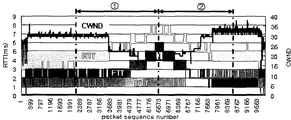
(그림 7) 수정된TCP Vegas에서의 순방향 지연 시 RTT와 CWND의 관계
