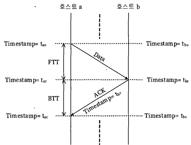
(그림 1) 종단간 순방향/역방향 전송 지연 측정 파라미터
