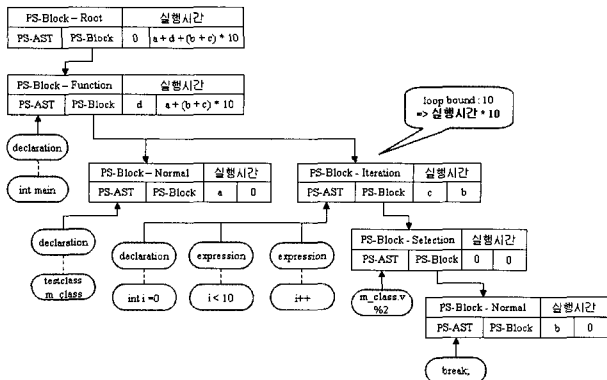
(그림 8) PS-Block Timing Model 구조
