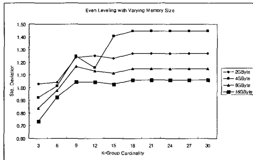
(그림 8) 플래시 메모리 크기에 대한 레벨링
