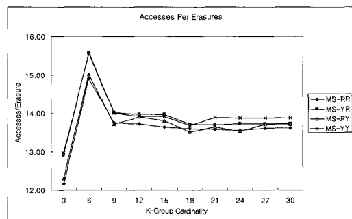
(그림 5) 최적 K값(세그먼트 소거 당 접근수)
