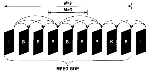
그림 1. 종속관계를 갖는 GOP 구조 예
