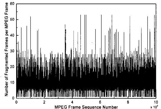
그림 11. MPEG4 프레임 크기 분포 예
