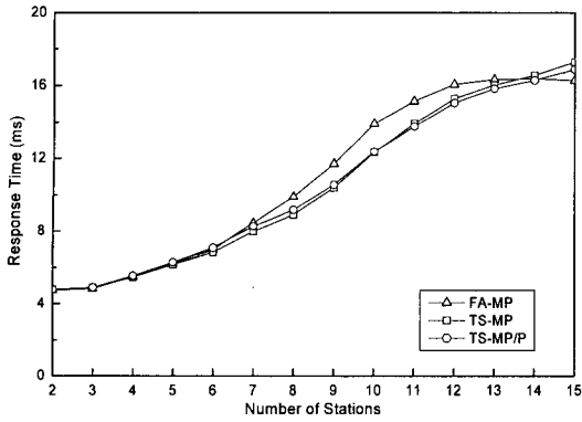
그림 12. 단말 수에 따른 전달시간
