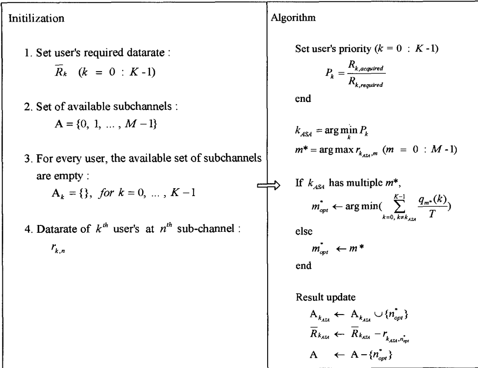
그림 4. ASA 알고리즘
