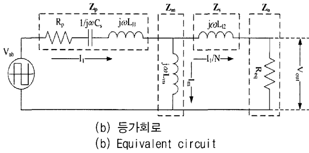
그림 3 무접점 변압기 적용 Full-bridge LLC 공진컨버터와 등가회로
