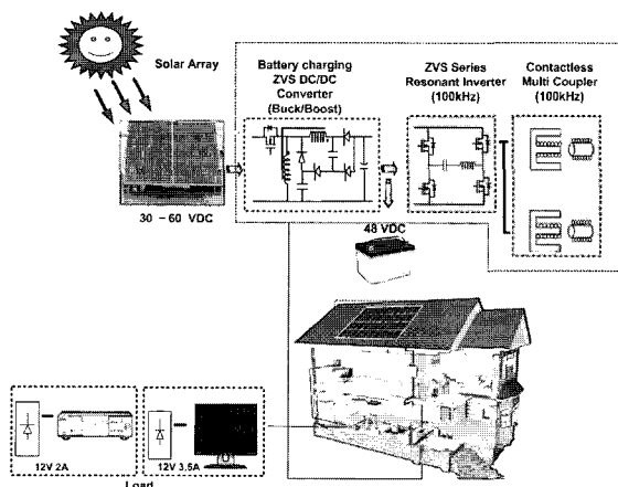
(b) 제안된 무접점 전원장치적용 태양광 발전 시스템 (b) The proposed photovoltaic power generation system using contactless power supply
