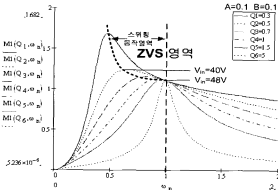
그림 4 무접점 변압기 적용 Full-bridge LLC 공진컨버터의 전압이득 특성 Fig. 4 Voltage gain characteristics of full-bridge LLC resonant converter using a contact-less transformer
