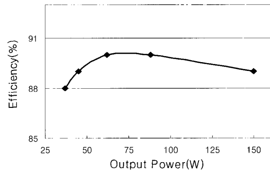
그림 7 부하출력 변화에 대한 효율특성
