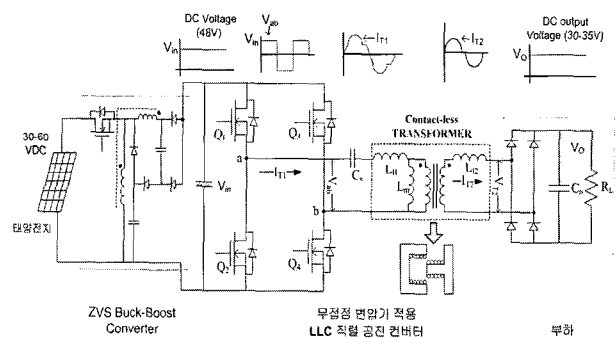
그림 5 태양광 발전 무접점 전원장치 적용 주회로도 Fig. 5 Main circuit of the contact-less power supply for photovoltaic power generation system
